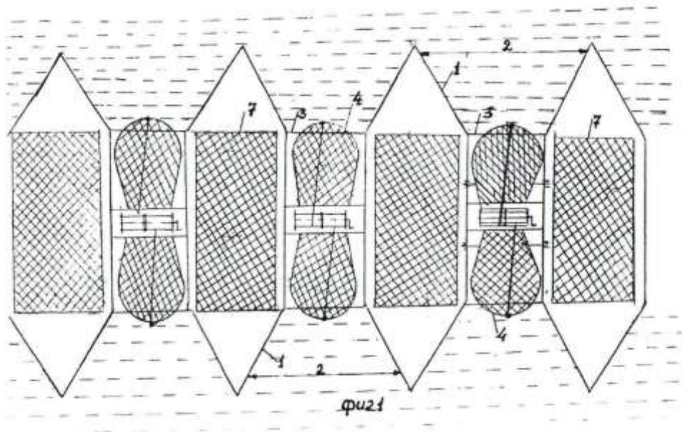
Рис. 3. Устройство для очистки водоемов от сине-зеленых водорослей
