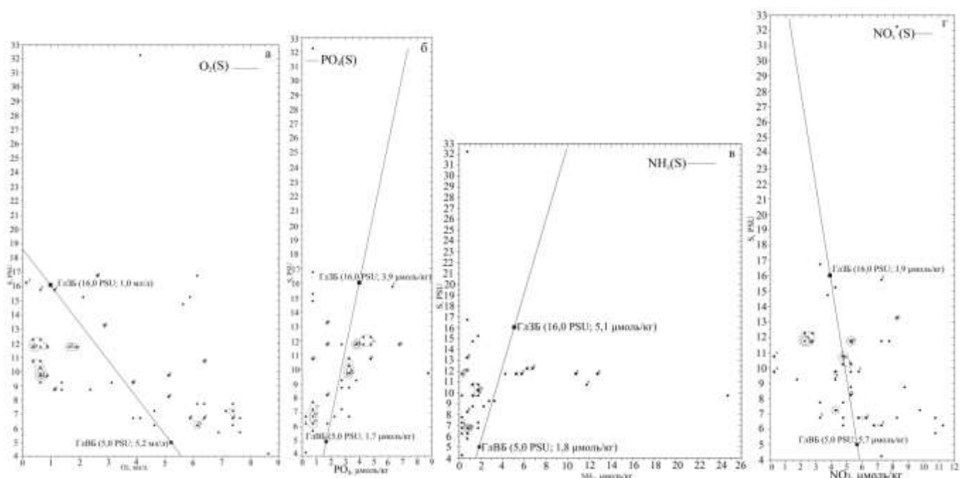
Рис. 3. Среднегодовые статистические S,O 2 - (а); S,PO 4 - (б); S,NH 4 - (в) и S,NO 3 - (г) диаграммы глубинных (ГлВБ и ГлЗБ) вод Балтийского моря в одноградусных трапециях, средние за 1900-2005 гг., по данным [1], рассчитанные по методике [2]
