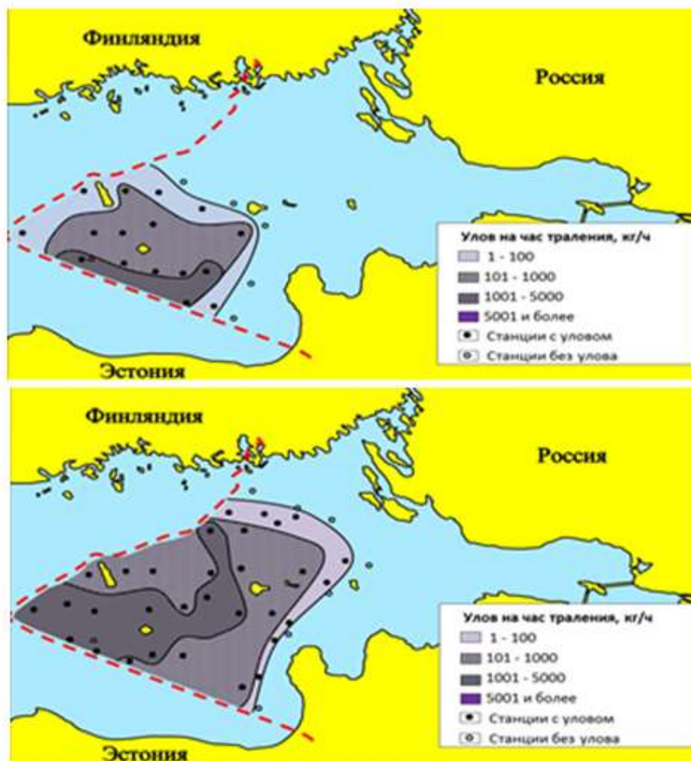
Рис. 4. Распределение шпрота в восточной части Финского залива по материалам промысловых уловов в октябре (А) и ноябре (Б) 2017 г., кг/час траления [11, с.40-46].
