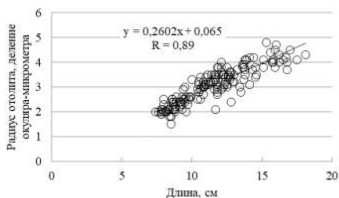
Рис. 2. Зависимость между радиусом отоликов и длиной корюшки рек бассейна Курицкого залива
